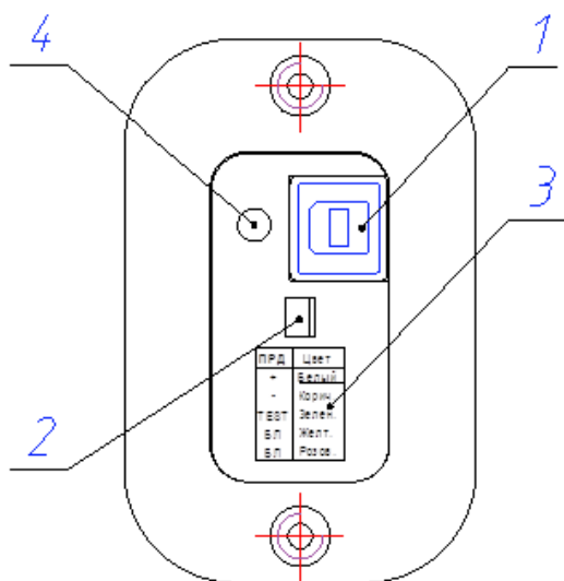
Рисунок 1.5 – Органы настройки блока ПРД извещателей «ТРЕЗОР-М»
