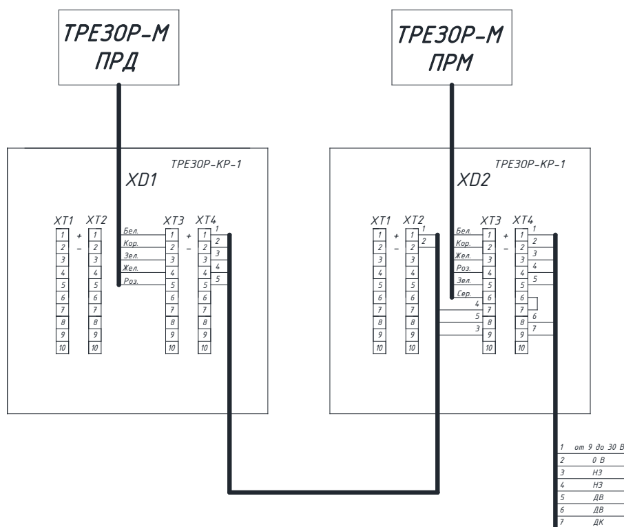
Рисунок 2.7 – Схема подключения извещателя при использовании распределительных коробок «ТРЕЗОР-КР-1» через блок ПРМ
