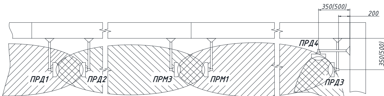
Рисунок 2.6 – Пример установки извещателя с применением выносных кронштейнов «Кронштейн 350» и «Кронштейн 500»
