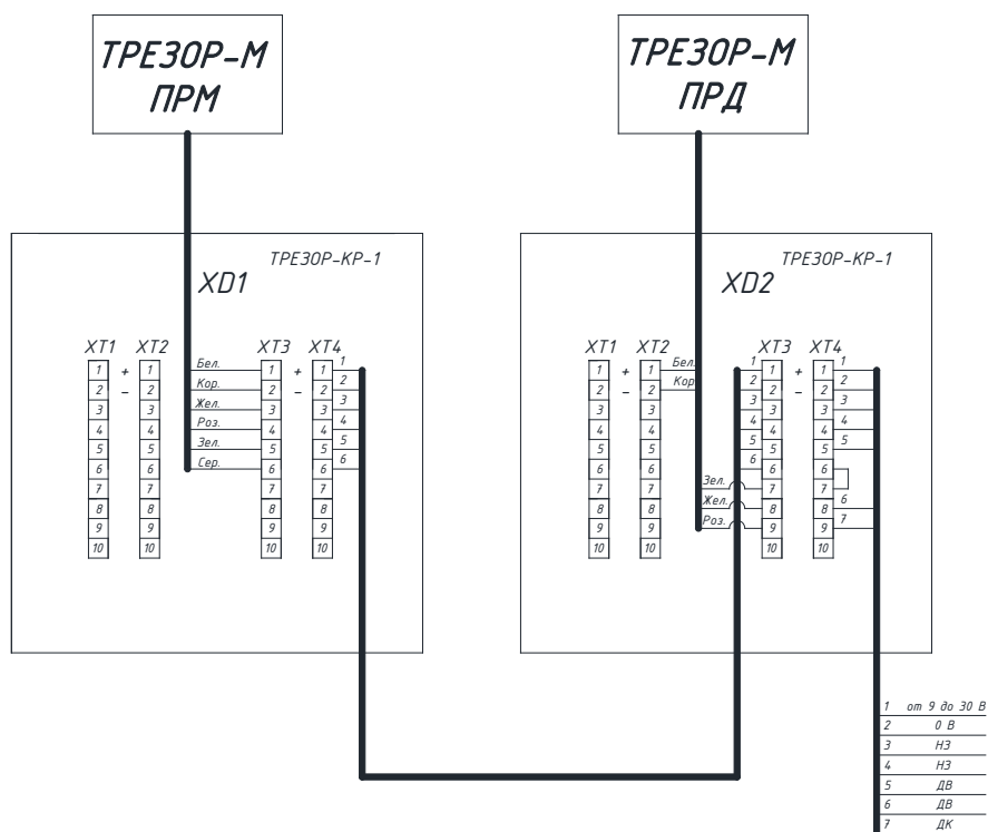
Рисунок 2.8 – Схема подключения извещателя при использовании распределительных коробок «ТРЕЗОР-КР-1» через блок ПРД
