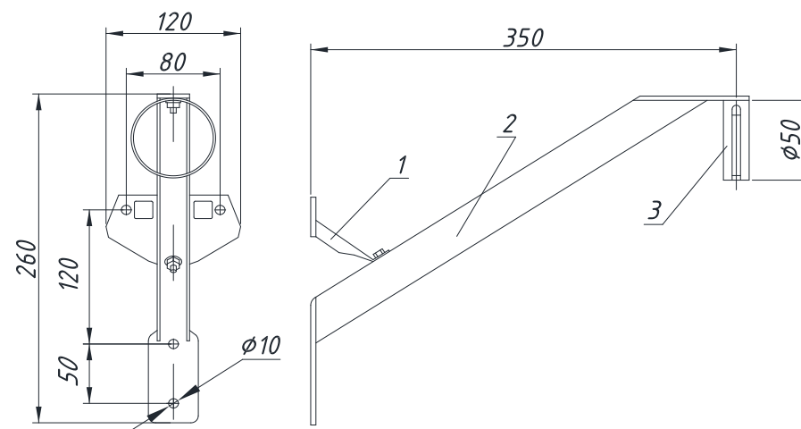
Рисунок 4.1 – Габаритные размеры и размеры для монтажа Изделия:
