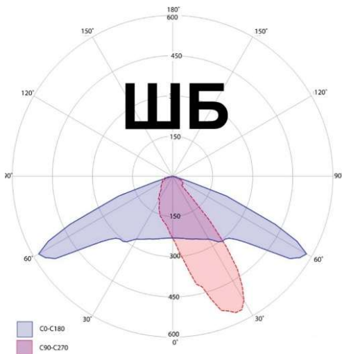
Рисунок 2- Диаграмма КСС ШБ
