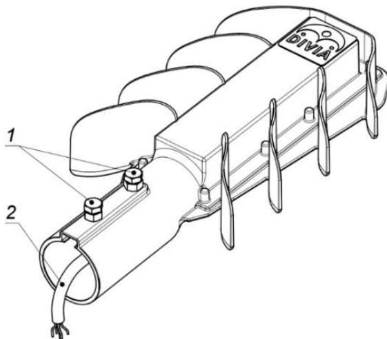
Рисунок 3 – Внешний вид изделия
