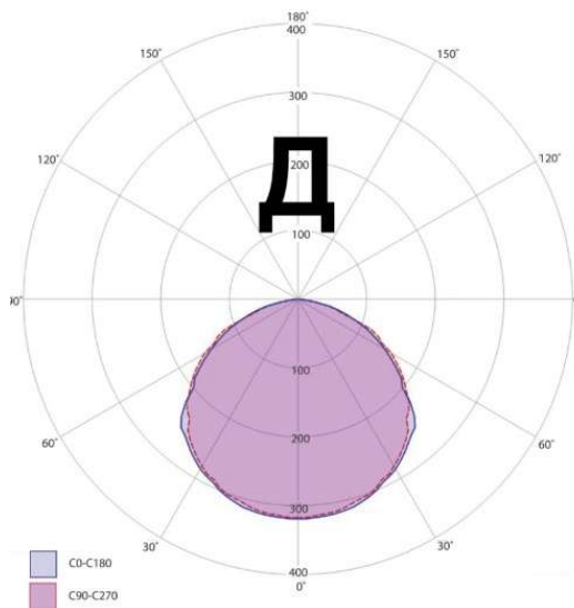
Рисунок 1- Диаграмма КСС Д
