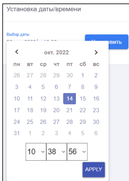
Рисунок 2.34 – Окно календаря
