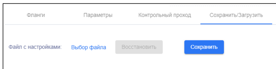
Рисунок 2.20 – Вкладка «Сохранить/Загрузить»
