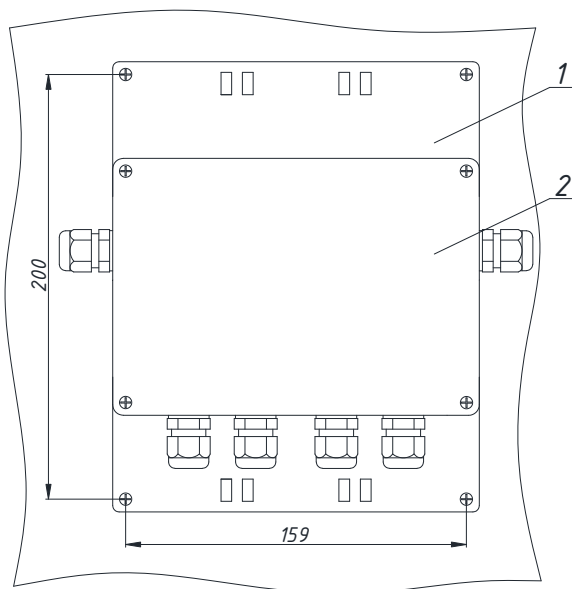
Рисунок 4 – Монтаж Изделия на стене.
