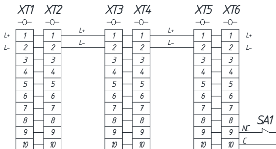
Рисунок 2 – Схема соединений
