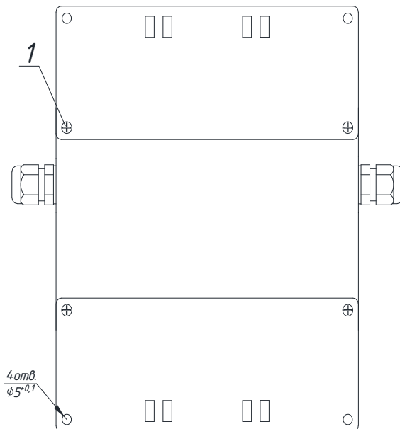
Рисунок 3 – Крепление кронштейнов к Изделию.
