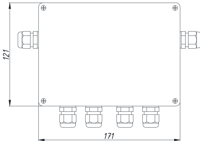
Рисунок 1 – Коробка распределительная КР-2. Внешний вид
