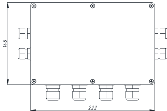
Рисунок 1.а – Коробка распределительная КР-3. Внешний вид
