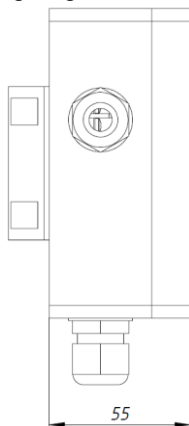
Рисунок 1.б - Коробка распределительная КР-2. Вид сбоку
