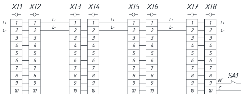
Рисунок 2 – Схема соединений
