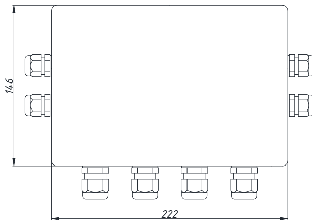
Рисунок 1 – Коробка распределительная КР-3. Внешний вид
